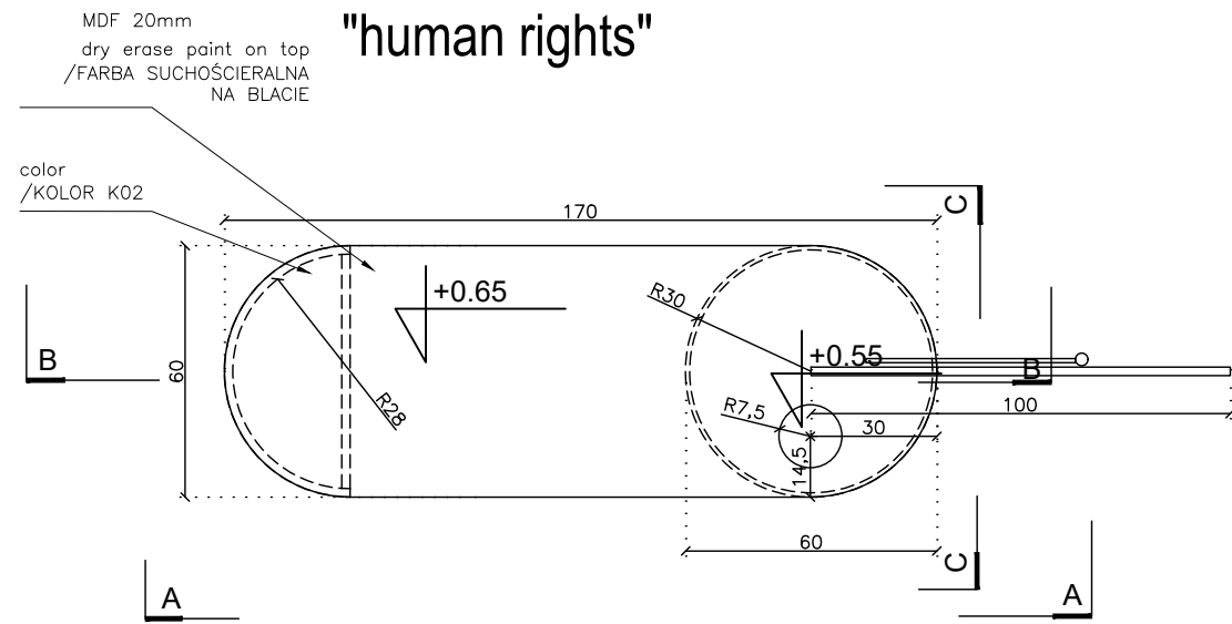
top view WIDOK Z GÓRY
