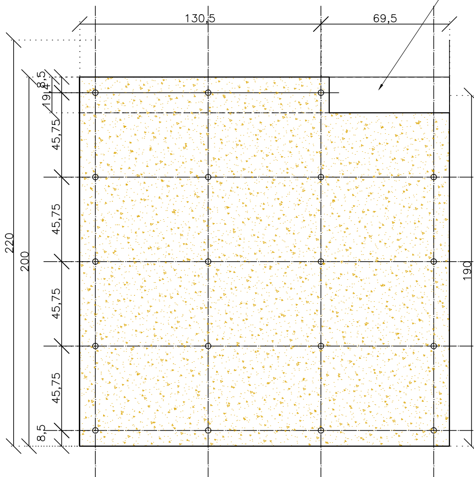
front view WIDOK Z PRZODU
