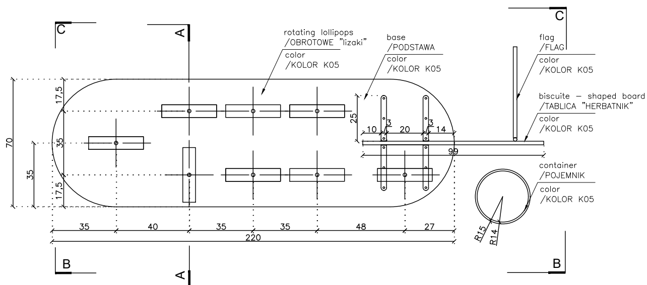
top view WIDOK Z GÓRY
